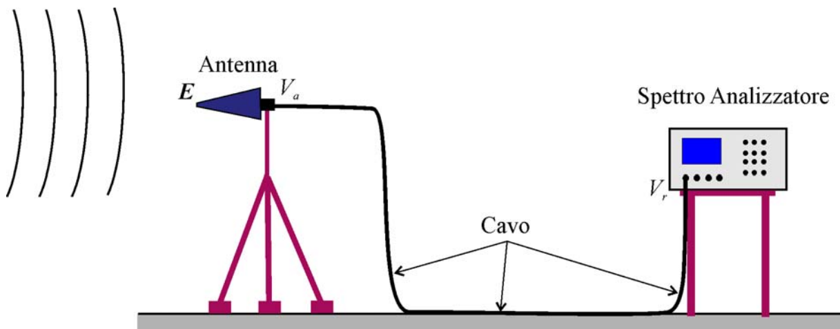
Figura 1- Schema di set-up di misura.
