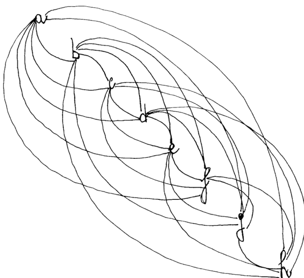
Figura 1: Un sistema di otto unità (o vertici) presenterà 256 gruppi possibili ( 2^8 ) e 56 cioè ( 8 \times 7 ) collegamenti (o bordi). Consideriamo ogni collegamento biunivoco e, nel caso rappresentato in figura, non tra gruppi (altrimenti sarebbe 256 \times 255 ). In qualsiasi punto può essere aggiunto un blocco di testo nuovo, un collegamento può essere interrotto o eliminato e un qualsiasi percorso è sempre tracciato e mantenuto in memoria dal sistema. In tal modo, considerando il raggruppamento insiemistico di due o più nodi si genera una progressione di raggruppamenti di ordini superiori, in cui rimangono sempre sotto controllo i vertici e i bordi: se ogni risultato generato dall'operazione 2^x=y , dove x è la quantità di elementi del sistema, si riscrive come esponente di 2, avremo la serie 2^y=z , 2^z=u , 2^u=r , ... . Teoricamente è sufficiente partire da almeno due elementi, per generare una progressione infinita. Un riferimento pratico può essere l'insieme di fonemi base di una lingua da cui si genera l'insieme infinito di catene fonemache potenziali. Inoltre per ogni gruppo basta applicare la formula n*(n-1) all'esponente o al risultato per sapere il numero dei collegamenti biunivoci possibili; banalmente il numero delle linee di collegamento sarà dato dalla formula (n*(n-1)) / 2 .
