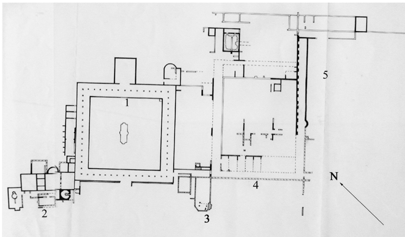
Fig. 1. Roma. Pineta di Castel Fusano. Villa di Plinio. Planimetria generale.
