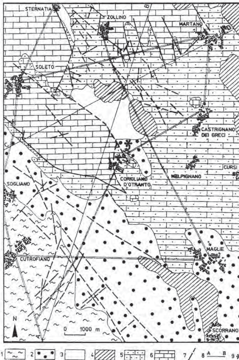
Fig. 1 - Carta geologica. 1) Depositi marini terrazzati; 2) Calcareniti di Gravina; 3) Sabbie di Uggiano; 4) Calcarenite di Andrano; 5) Pietra leccese; 6) Calcarea di Altamura; 7) faglia; 8) traccia sezione; 9) pozzo di cui si riportano la stratigrafia ed i carotaggi multiparametrici (Cfr. Fig. 6).
