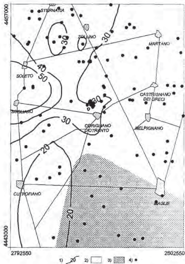
Fig. 10 - Distribuzione dell'ammoniaca e dei nitrati. 1) isolina \text{NO}_3^- ( \text{mg}/\text{l} ); 2) 0,05-0,5 \text{ mg}/\text{l} di \text{NH}_4^+ ; 3) >0,5 \text{ mg}/\text{l} di \text{NH}_4^+ ; 4) pozzo di misura.
