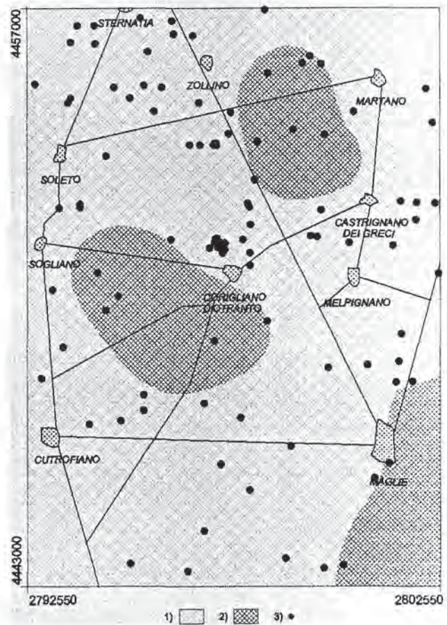
Fig. 7 - Distribuzione della soggiacenza (m s.l.m.); 1) 50-100m; 2) >100m; 3) pozzo di misura.
