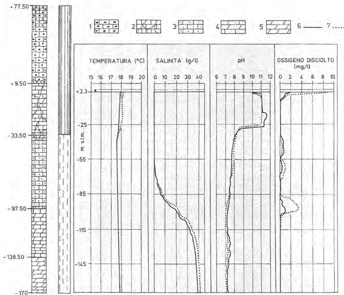
Fig. 6 - Pozzo C49; stratigrafia, tipica dell'area campione, ed andamento con la profondità di alcuni parametri chimico-fisici delle acque sotterranee dell'area di studio. 1) calcareniti con intercalazioni sabbioso-limose (Calcareniti di Gravina); 2) calcari micritici e calcari dolomitici a luoghi fratturati (Calcarenite di Andrano); 3) calcareniti tufacee con livelli macrofossiliferi (Pietra leccese); 4) calcari dolomitici e dolomie (Calcare di Altamura); 5) dolomie (Calcare di Altamura); carotaggio multiparametrico 6) del 16/04/1996 e del 7) del 04/11/1996.
