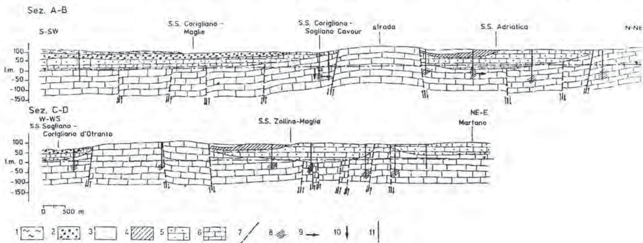
Fig. 2 - Sezioni Idrogeologiche. 1) Depositi marini terrazzati; 2) Calcareniti di Gravina; 3) Sabbie di Uggiano; 4) Calcareniti di Andrano; 5) Pietra leccese; 6) Calcare di Altamura; 7) faglia; 8) rinvenimento idrico; Determinazione mediante traccianti della 9) direzione prevalente della velocità di filtrazione e della 10) corrente idrica verticale; 11) pozzo.
