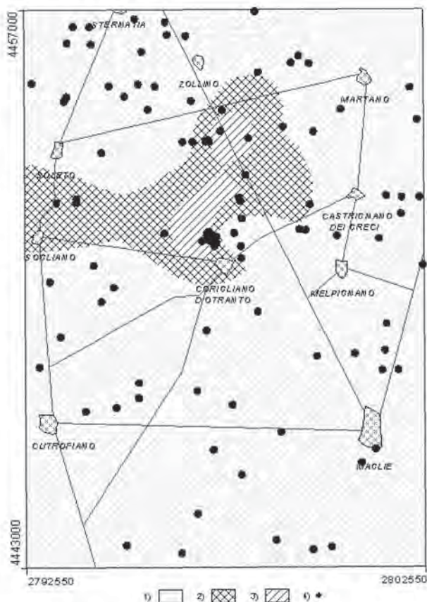
Fig. 9 - Distribuzione della Conducibilità elettrica delle acque sotterranee ad Aprile 1997 ( \mu\text{S}/\text{cm} a 25^\circ\text{C} ). 1) 600-700; 2) 700-800; 3) >800 ; 4) pozzo di misura.
