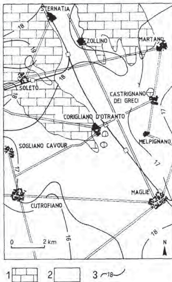
Fig. 3 - Andamento della temperatura nelle acque sotterranee a livello del mare (ricostruito mediante carotaggi della temperatura idrica). 1) Basamento mesozoico; 2) Depositi miocenici-pleistocenici; 3) Isotherma ( ^{\circ}\text{C} ).
