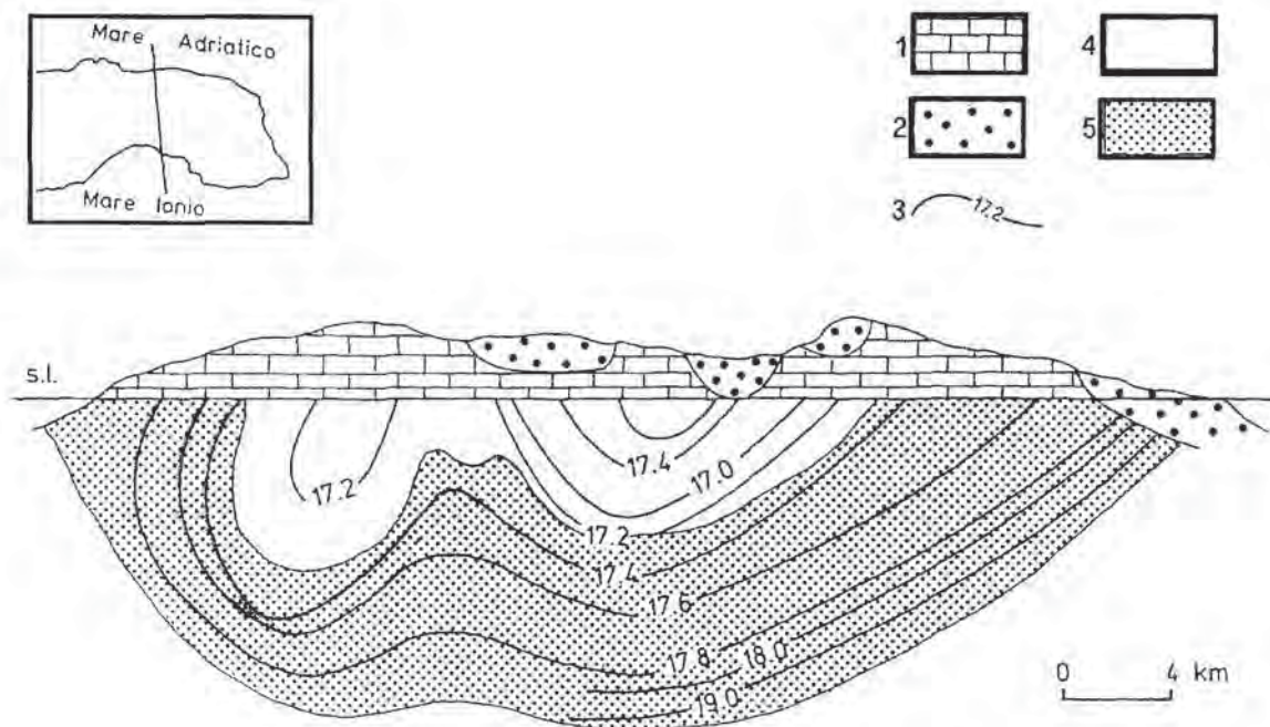
Fig. 4 - Distribuzione verticale della temperatura idrica nell'acquifero profondo (da Tulipano & Fidelibus, 1988, modificata). 1) Basamento mesozoico; 2) Depositi miocenici-pleistocenici; 3) Isotherma ( ^{\circ}\text{C} ); Acque sotterranee 4) dolci e 5) saline.
