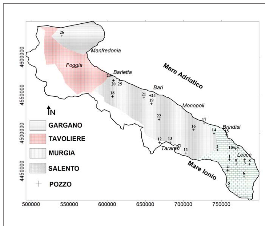
Figura 1. Principali strutture idrogeologiche pugliesi e ubicazione dei pozzi di monitoraggio piezometrico
