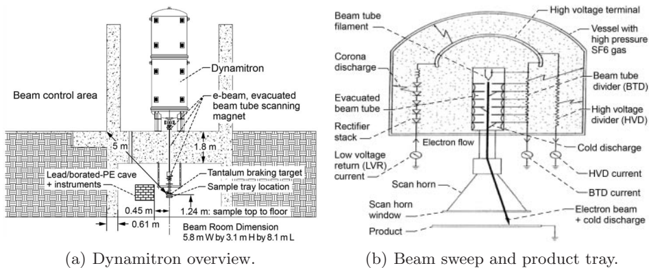
Fig. 2. – Schematic of Dynamitron.
