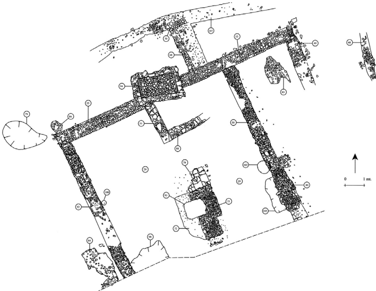
Fig. 4. Settore 2. Planimetria.
