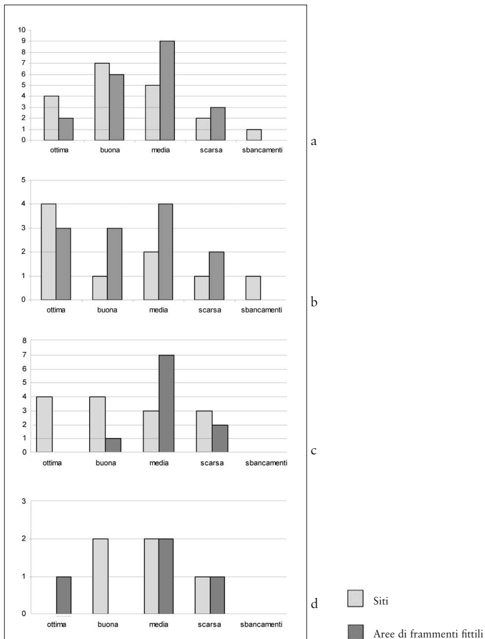
Fig. 3 – Roccella. Tipologia dei rinvenimenti per classi di visibilità del suolo: a) Terrazzi marini di I ordine; b) Trubi; c) fasce detritiche; d) Fm. Terravecchia.
